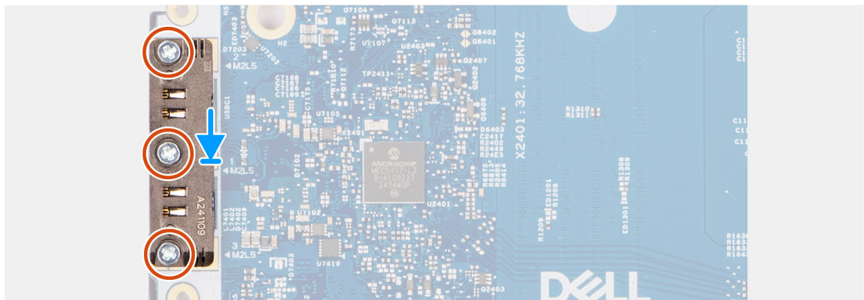
Ilustración 49. Instalación del módulo USB tipo C
