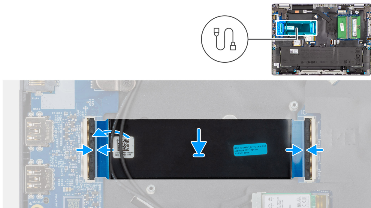
Ilustración 39. Instalación de la placa de I/O
