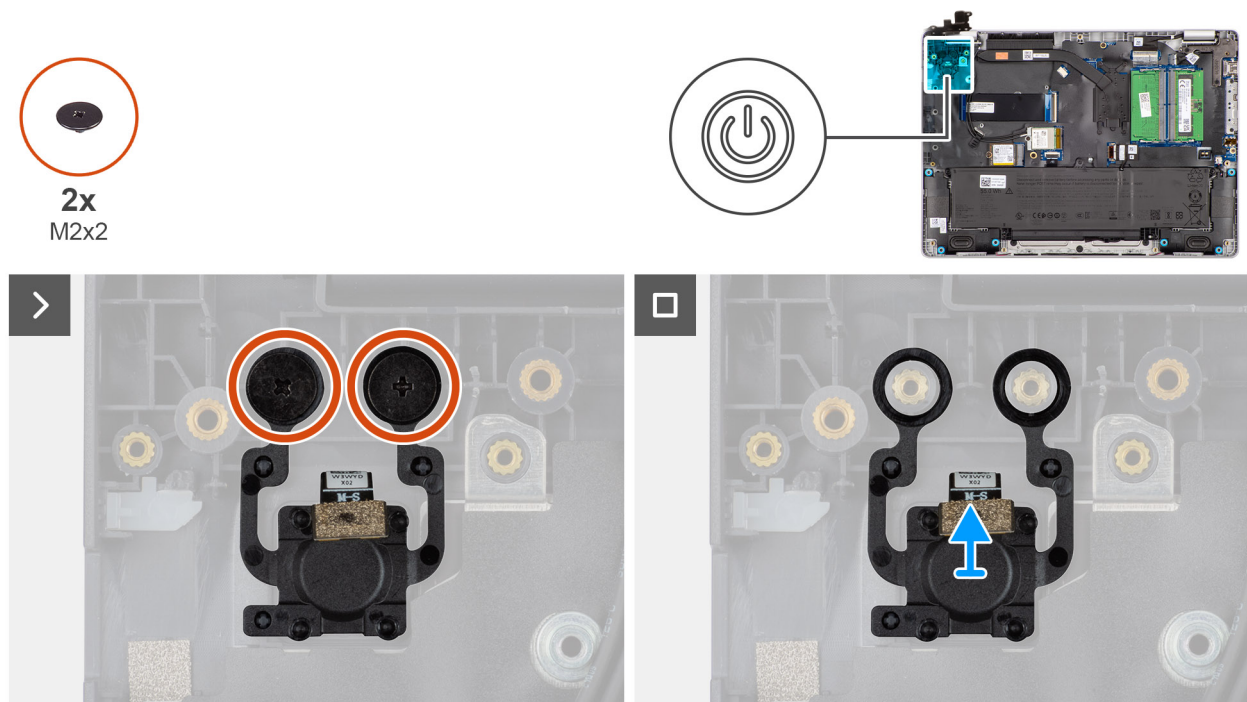
Ilustración 40. Extracción del botón de encendido con lector de huellas digitales
