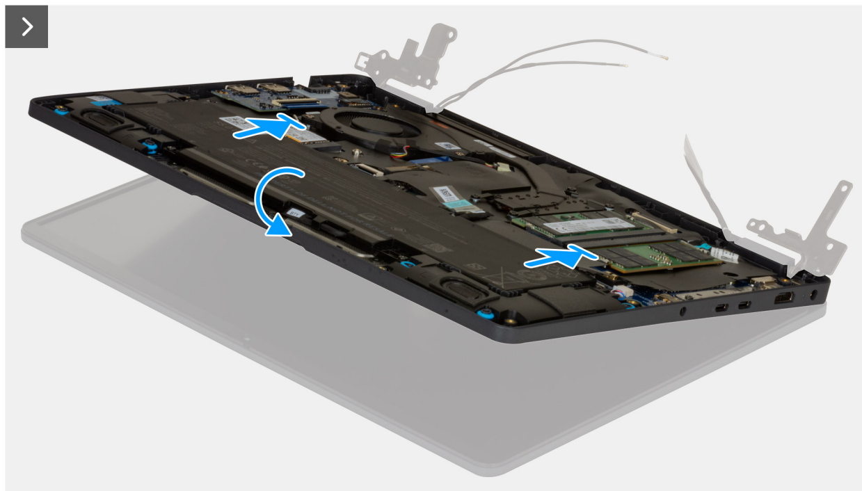
Ilustración 65. Instalación del ensamblaje de la pantalla
