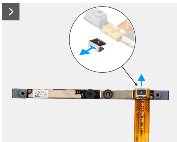
Ilustración 82. Extracción de la cámara
