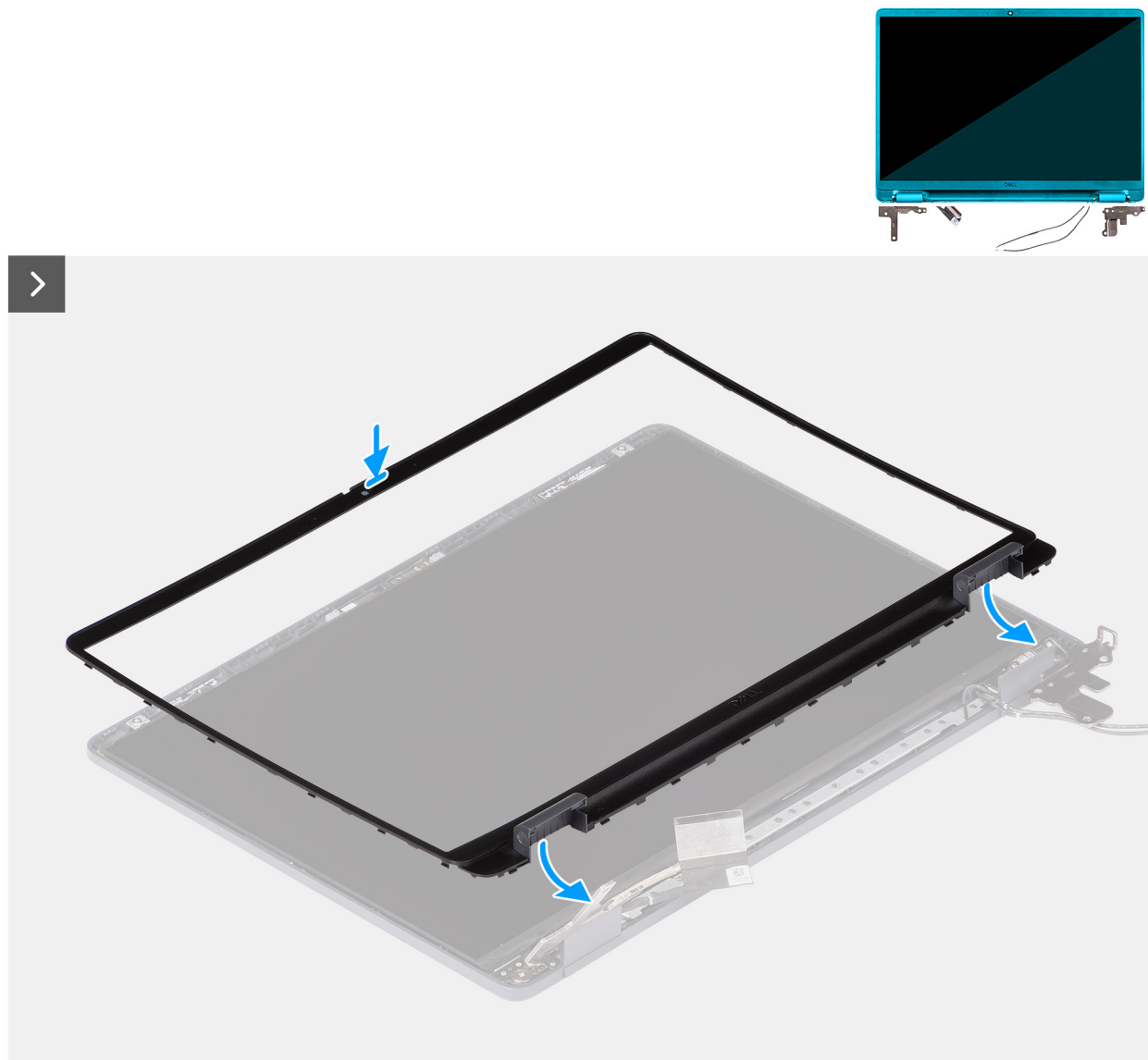
Ilustración 72. Instalación del bisel de la pantalla
