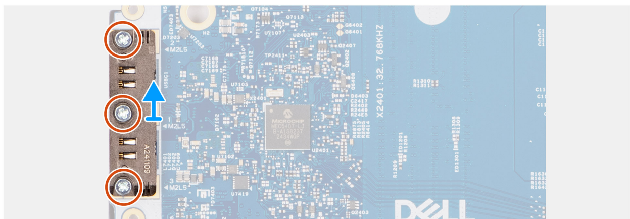
Ilustración 48. Extracción del módulo USB tipo C
