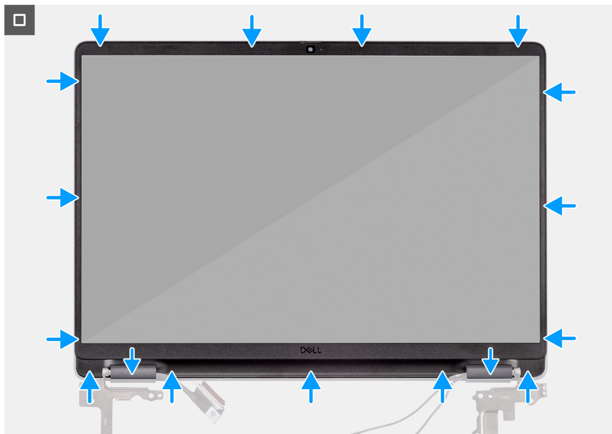
Ilustración 73. Instalación del bisel de la pantalla
