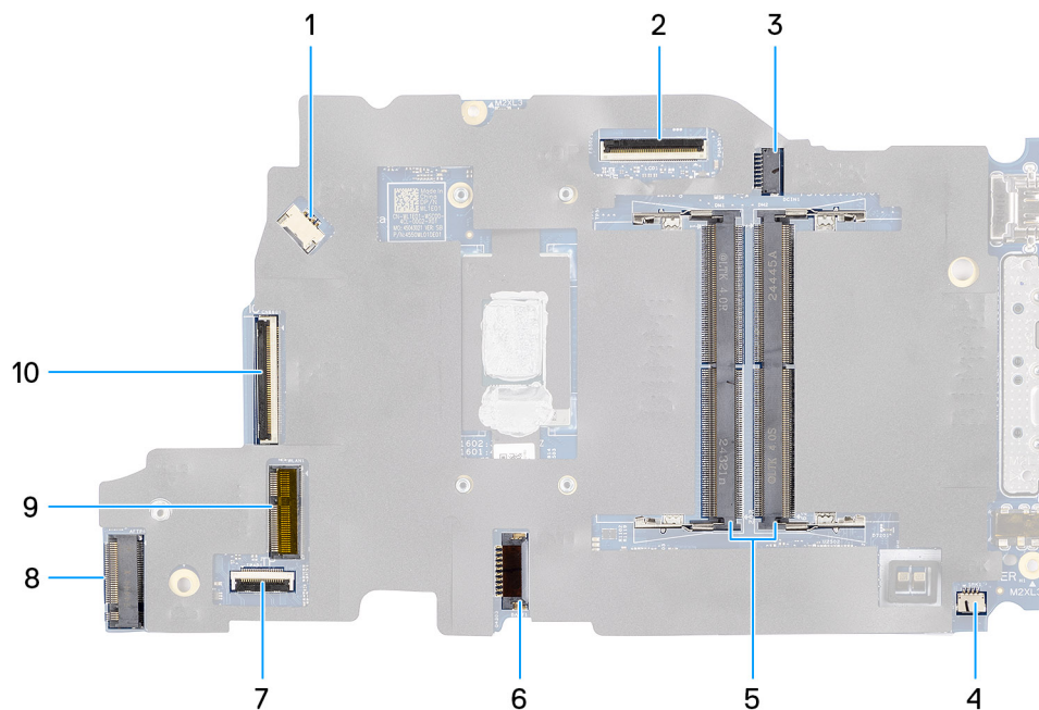
Ilustración 45. Conectores de la tarjeta madre
