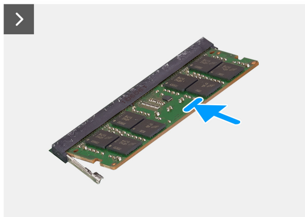
Ilustración 22. Instalación del módulo de memoria
