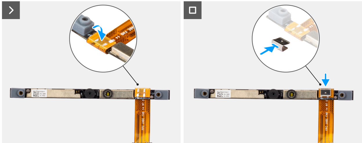
Ilustración 83. Instalación de la cámara
