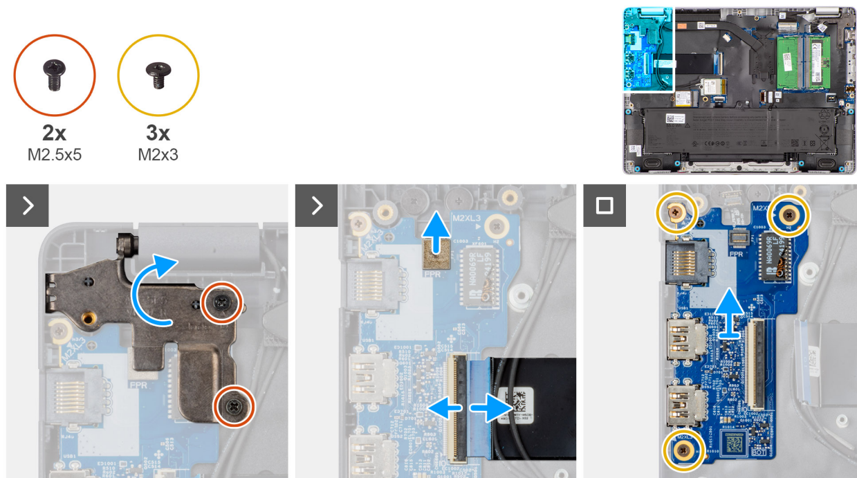
Ilustración 36. Extracción de la placa de I/O
